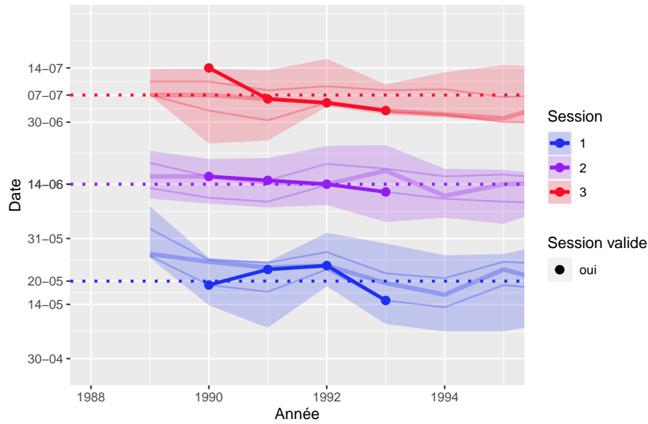
Figure 2: Les dates des 3 sessions sélectionnées pour la station 13a. Les lignes pointillées représentent les dates de références pour la station calculer à partir des dates locales de session. Les points de couleur (bleu pour la session 1, violet pour la session 2 et rouge pour la session 3) indiquent les sessions concernées pour l'analyse des indicateurs. En couleur pale est indiqué la distribution des dates des sessions à l'échelle nationale (en gras la médiane, en trait fin les 50% autour de la médiane et en ombré la zone des 95%)
