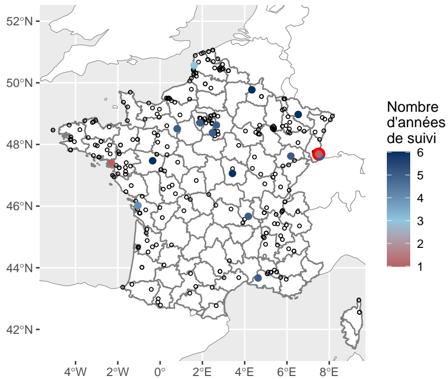
Figure 1: Localisation de la stations 13a en rouge et des stations de même type en dégradé de bleu présentant le nombre d'année de données disponibles pour la comparaison. Les stations notées par un petit cercle vide sont les stations qui ne sont pas utilisables pour caractériser la référence nationale
