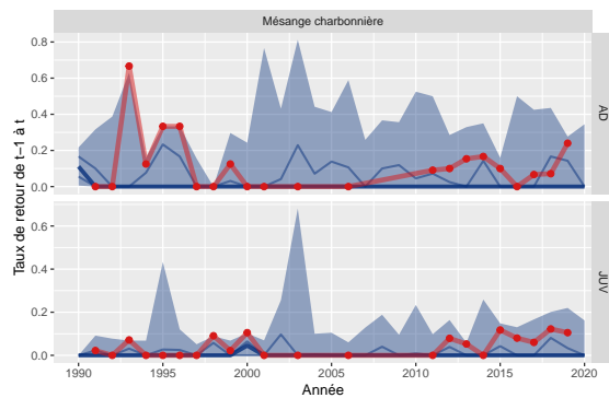
Figure 53: Variation du taux de retour de Mésange charbonnière pour la station 12 comparée aux STOC-Capture de type terrestre (n=259)
