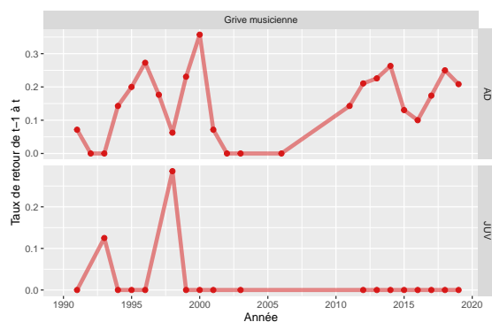
Figure 51: Variation du taux de retour de Grive musicienne pour la station 12 comparée aux STOC-Capture de type terrestre (n=230)
