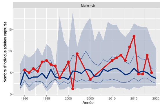
Figure 7: Variation du nombre d'adultes capturés de Merle noir pour le station 12 comparé aux STOC-Capture de type terrestre (n=260)
