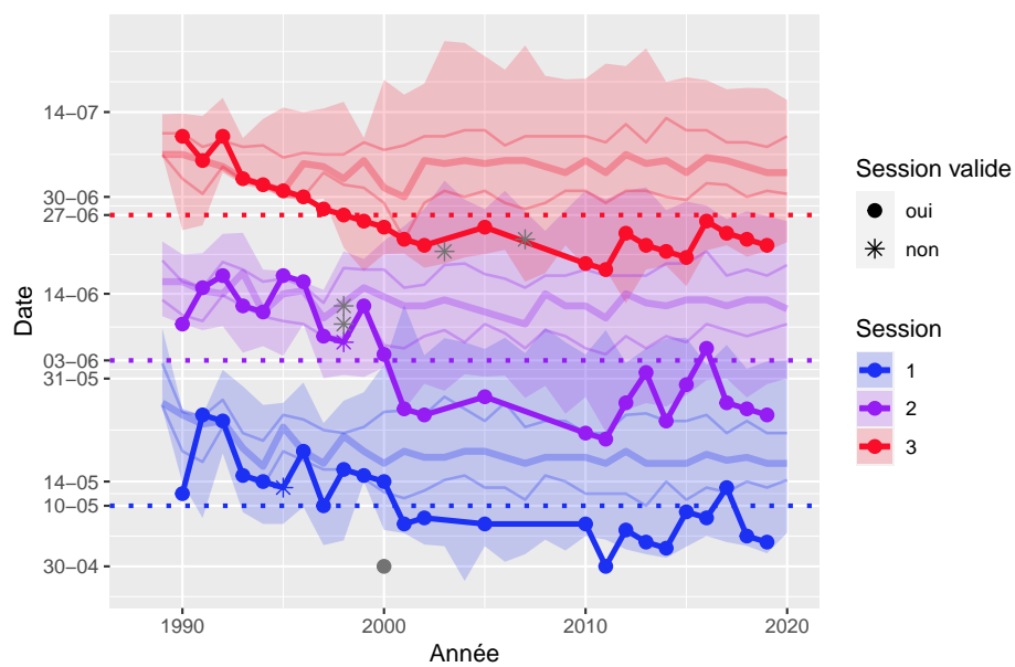
Figure 2: Les dates des 3 sessions sélectionnées pour la station 12. Les lignes pointillées représentent les dates de références pour la station calculer à partir des dates locales de session. Les points de couleur (bleu pour la session 1, violet pour la session 2 et rouge pour la session 3) indiquent les sessions concernées pour l'analyse des indicateurs. En couleur pale est indiqué la distribution des dates des sessions à l'échelle nationale (en gras la médiane, en trait fin les 50% autour de la médiane et en ombré la zone des 95%)
