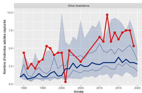
Figure 8: Variation du nombre d'adultes capturés de Grive musicienne pour le station 12 comparé aux STOC-Capture de type terrestre (n=230)
