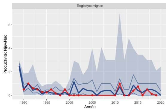
Figure 41: Variation de la productivité de Troglydte mignon pour la station 12 comparée aux STOC-Capture de type terrestre (n=230)
