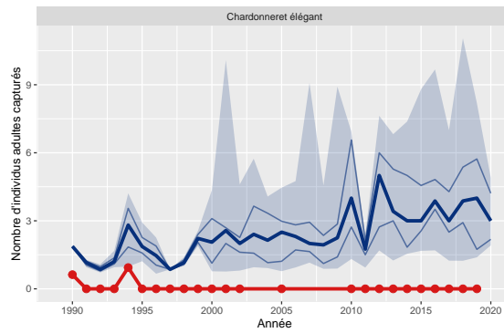
Figure 32: Variation du nombre d'adultes capturés de Chardonneret élégant pour le station 12 comparé aux STOC-Capture de type terrestre (n=103)
