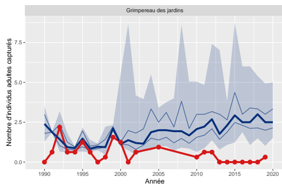
Figure 18: Variation du nombre d'adultes capturés de Grimpereau des jardins pour le station 12 comparé aux STOC-Capture de type terrestre (n=187)
