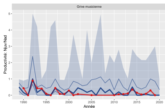
Figure 37: Variation de la productivité de Grive musicienne pour la station 12 comparée aux STOC-Capture de type terrestre (n=230)
