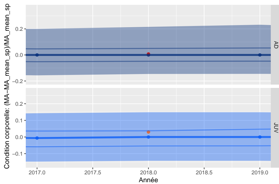
Figure 42: Variation de la condition corporelle globale pour la station 12. En bleu, la variation des quantiles de l'indicateur national (médiane, 50% et 95%) pour les stations de type terrestre, en rouge et orange la variation pour la station 12
