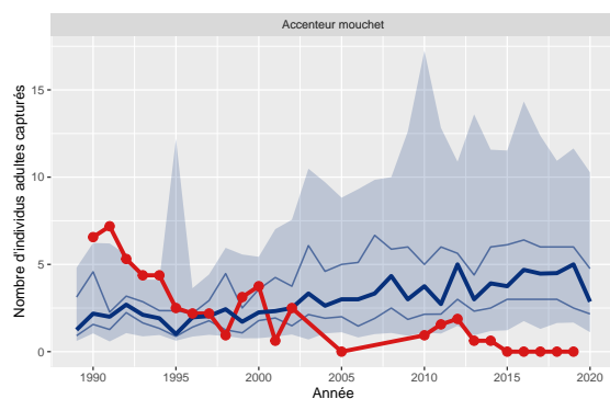
Figure 11: Variation du nombre d'adultes capturés de Accenteur mouchet pour le station 12 comparé aux STOC-Capture de type terrestre (n=216)
