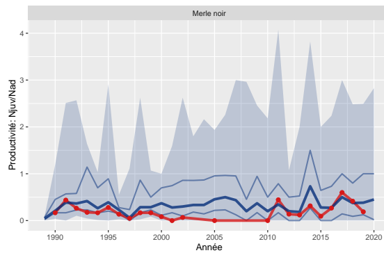
Figure 36: Variation de la productivité de Merle noir pour la station 12 comparée aux STOC-Capture de type terrestre (n=260)
