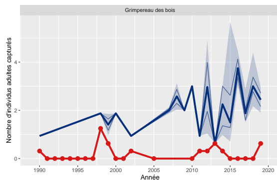
Figure 24: Variation du nombre d'adultes capturés de Grimpereau des bois pour le station 12 comparé aux STOC-Capture de type terrestre (n=24)
