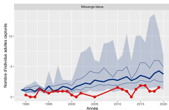
Figure 17: Variation du nombre d'adultes capturés de Mésange bleue pour le station 12 comparé aux STOC-Capture de type terrestre (n=243)
