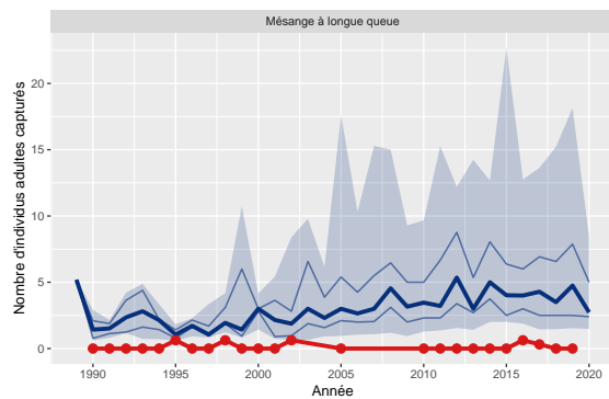
Figure 28: Variation du nombre d'adultes capturés de Mésange à longue queue pour le station 12 comparé aux STOC-Capture de type terrestre (n=209)
