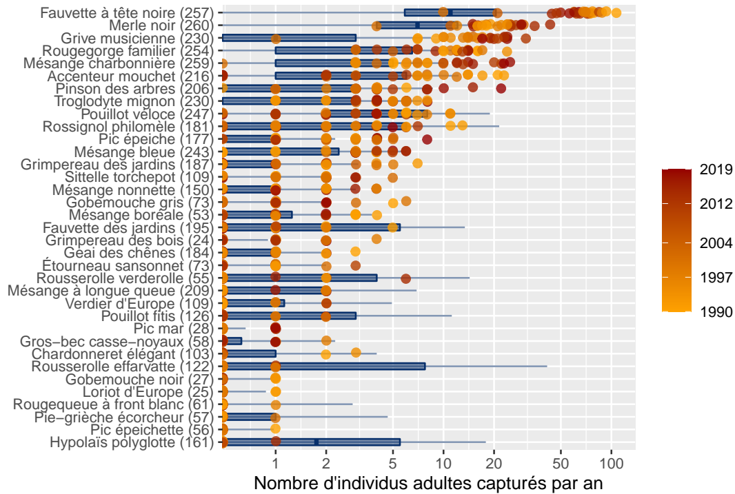
Figure 4: Nombre d'adulte capturés par espèce sur la station 12, les points dégradés du jaune au rouge (correspondant aux années) représentent les données locales, les boîtes à moustaches bleues représentent la distribution nationale de ces captures sur les stations de type terrestre et qui capturent l'espèce. Le nombre de station qui capture l'espèce est noté entre parenthèse
