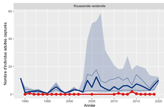
Figure 27: Variation du nombre d'adultes capturés de Rousserolle verderolle pour le station 12 comparé aux STOC-Capture de type terrestre (n=55)
