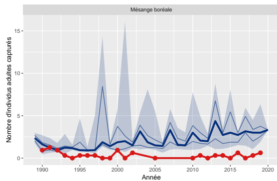
Figure 22: Variation du nombre d'adultes capturés de Mésange boréale pour le station 12 comparé aux STOC-Capture de type terrestre (n=53)
