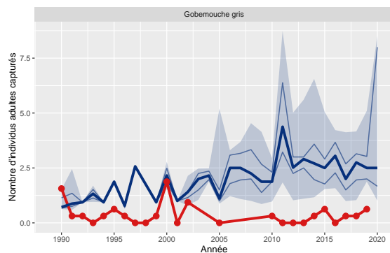
Figure 21: Variation du nombre d'adultes capturés de Gobemouche gris pour le station 12 comparé aux STOC-Capture de type terrestre (n=73)
