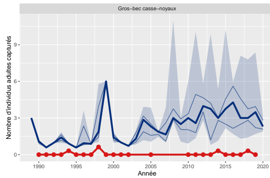
Figure 33: Variation du nombre d'adultes capturés de Gros-bec casse-noyaux pour le station 12 comparé aux STOC-Capture de type terrestre (n=58)
