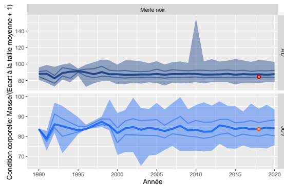
Figure 44: Variation de la condition corporelle des Merle noir pour le station 12 comparée aux STOC-Capture de type terrestre (n=260)
