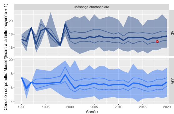
Figure 47: Variation de la condition corporelle des Mésange charbonnière pour le station 12 comparée aux STOC-Capture de type terrestre (n=259)
