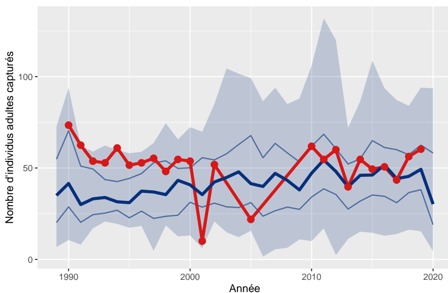
Figure 5: Variation du nombre d'adultes capturés pour la station 12 comparée aux STOC-Capture de type terrestre.
