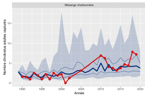
Figure 10: Variation du nombre d'adultes capturés de Mésange charbonnière pour le station 12 comparé aux STOC-Capture de type terrestre (n=259)
