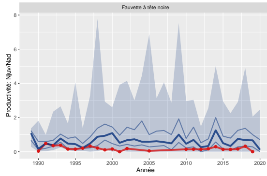
Figure 35: Variation de la productivité de Fauvette à tête noire pour la station 12 comparée aux STOC-Capture de type terrestre (n=257)
