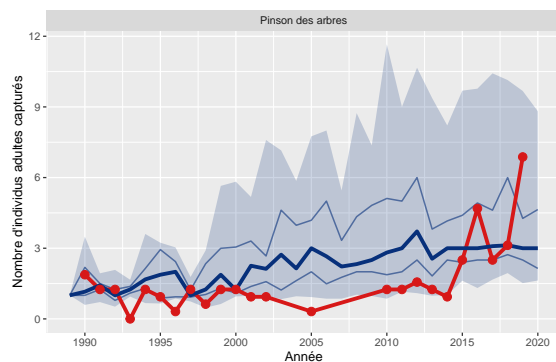
Figure 12: Variation du nombre d'adultes capturés de Pinson des arbres pour le station 12 comparé aux STOC-Capture de type terrestre (n=206)
