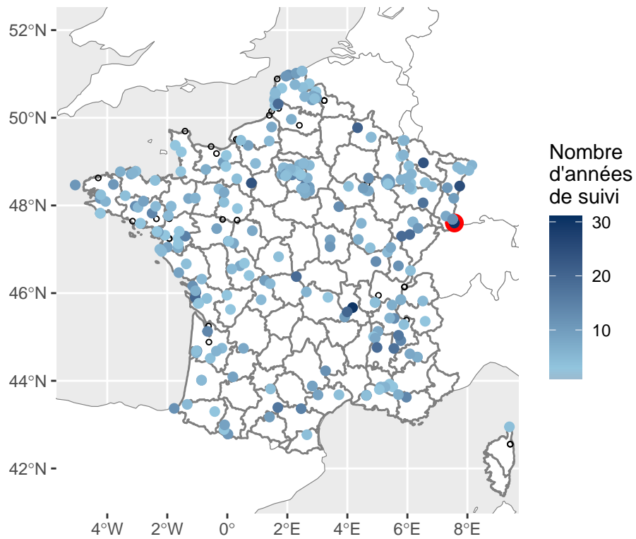
Figure 1: Localisation de la stations 12 en rouge et des stations de même type en dégradé de bleu présentant le nombre d'année de données disponibles pour la comparaison. Les stations notées par un petit cercle vide sont les stations qui ne sont pas utilisables pour caractériser la référence nationale
