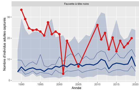
Figure 6: Variation du nombre d'adultes capturés de Fauvette à tête noire pour le station 12 comparé aux STOC-Capture de type terrestre (n=257)
