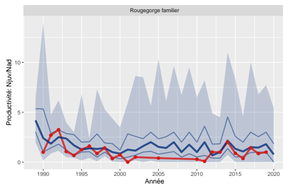
Figure 38: Variation de la productivité de Rougegorge familier pour la station 12 comparée aux STOC-Capture de type terrestre (n=254)
