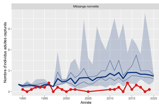
Figure 20: Variation du nombre d'adultes capturés de Mésange nonnette pour le station 12 comparé aux STOC-Capture de type terrestre (n=150)
