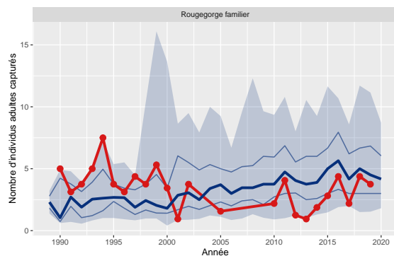
Figure 9: Variation du nombre d'adultes capturés de Rougegorge familier pour le station 12 comparé aux STOC-Capture de type terrestre (n=254)
