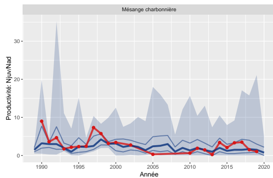
Figure 39: Variation de la productivité de Mésange charbonnière pour la station 12 comparée aux STOC-Capture de type terrestre (n=259)
