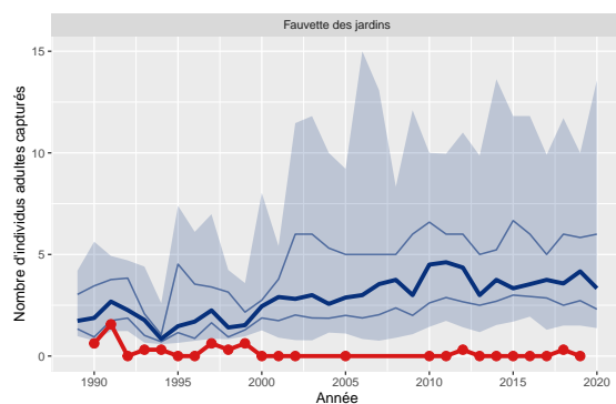
Figure 23: Variation du nombre d'adultes capturés de Fauvette des jardins pour le station 12 comparé aux STOC-Capture de type terrestre (n=195)
