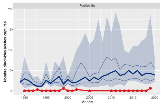
Figure 31: Variation du nombre d'adultes capturés de Pouillot fitis pour le station 12 comparé aux STOC-Capture de type terrestre (n=126)
