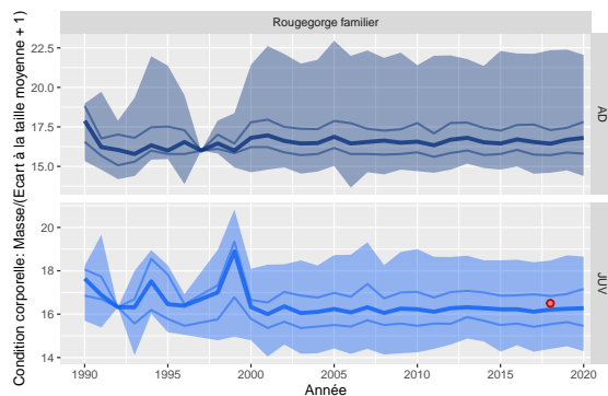
Figure 46: Variation de la condition corporelle des Rougegorge familier pour le station 12 comparée aux STOC-Capture de type terrestre (n=254)
