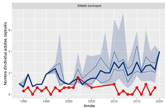
Figure 19: Variation du nombre d'adultes capturés de Sittelle torchepot pour le station 12 comparé aux STOC-Capture de type terrestre (n=109)
