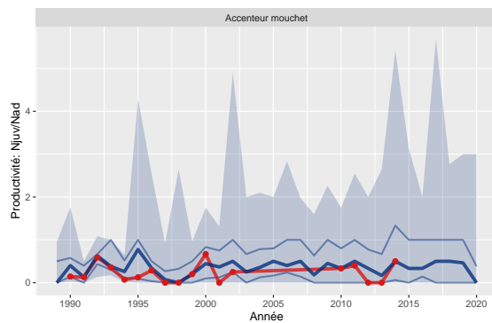
Figure 40: Variation de la productivité de Accenteur mouchet pour la station 12 comparée aux STOC-Capture de type terrestre (n=216)
