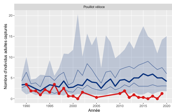
Figure 14: Variation du nombre d'adultes capturés de Pouillot véloce pour le station 12 comparé aux STOC-Capture de type terrestre (n=247)
