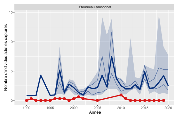
Figure 26: Variation du nombre d'adultes capturés de Étourneau sansonnet pour le station 12 comparé aux STOC-Capture de type terrestre (n=73)
