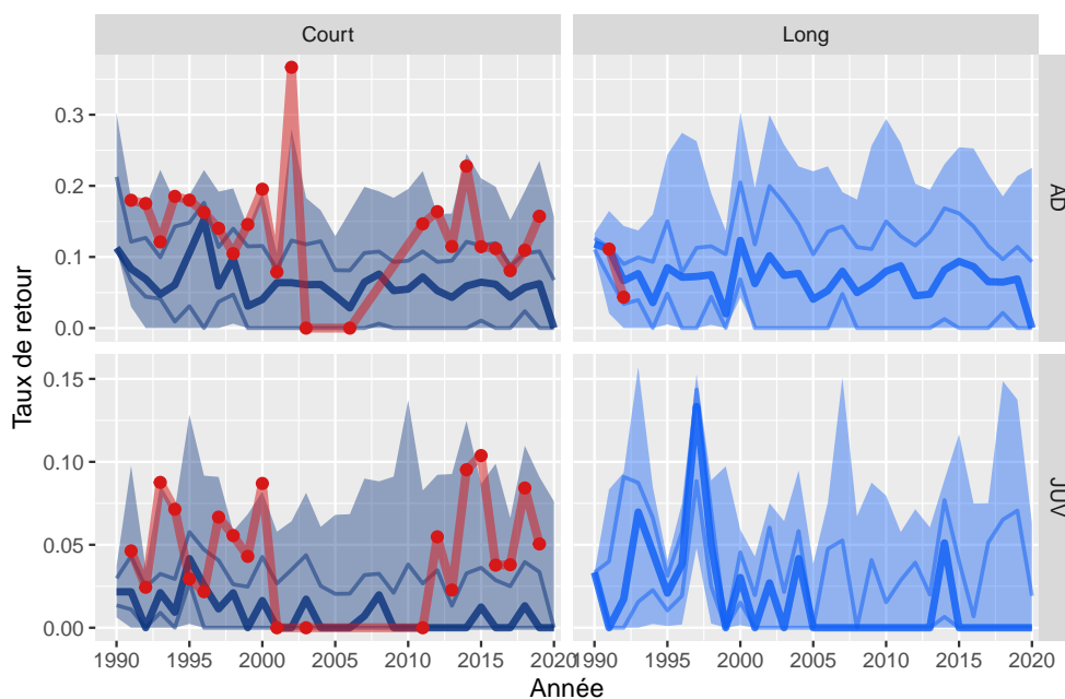
Figure 48: Variation du taux de retour sur l'ensemble des espèces pour la station 12. Le taux de retour de l'année t est la proportion des individus qui sont revus à l'année t + 1 . En bleu, la variation des quantiles de l'indicateur national (médiane, 50% et 95%) des stations de type terrestre, en rouge et orange la variation pour la station 12.
