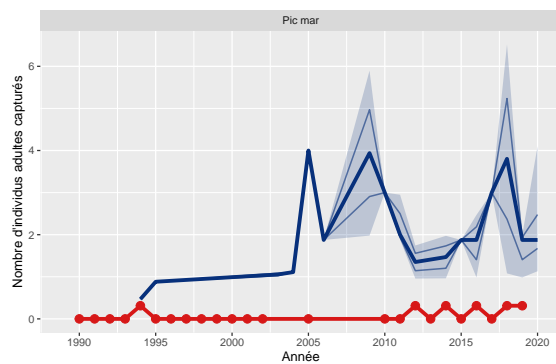
Figure 30: Variation du nombre d'adultes capturés de Pic mar pour le station 12 comparé aux STOC-Capture de type terrestre (n=28)
