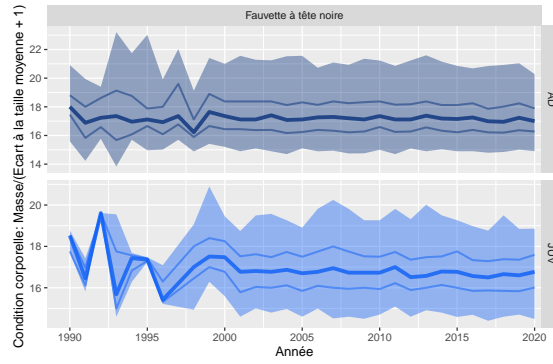
Figure 43: Variation de la condition corporelle des Fauvette à tête noire pour le station 12 comparée aux STOC-Capture de type terrestre (n=257)
