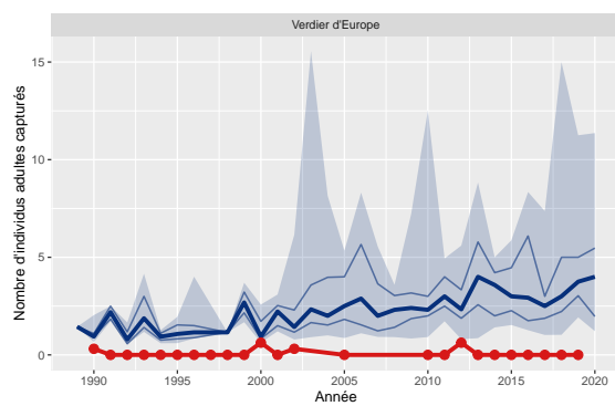
Figure 29: Variation du nombre d'adultes capturés de Verdier d'Europe pour le station 12 comparé aux STOC-Capture de type terrestre (n=109)
