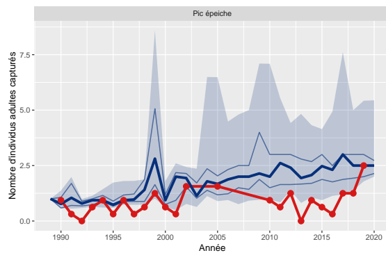
Figure 16: Variation du nombre d'adultes capturés de Pic épeiche pour le station 12 comparé aux STOC-Capture de type terrestre (n=177)
