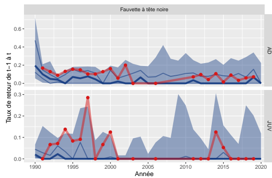
Figure 49: Variation du taux de retour de Fauvette à tête noire pour la station 12 comparée aux STOC-Capture de type terrestre (n=257)
