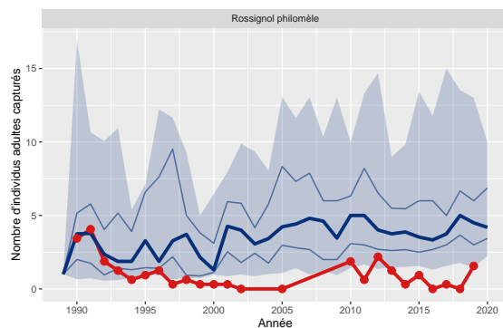
Figure 15: Variation du nombre d'adultes capturés de Rossignol philomèle pour le station 12 comparé aux STOC-Capture de type terrestre (n=181)
