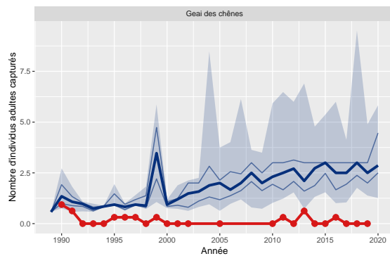
Figure 25: Variation du nombre d'adultes capturés de Geai des chênes pour le station 12 comparé aux STOC-Capture de type terrestre (n=184)
