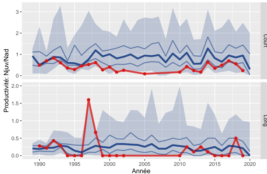
Figure 34: Variation de la productivité globale pour la station 12. En bleu, la variation nationale des quantiles de l'indicateur (médiane, 50% et 95%) pour les station de type terrestre, en rouge la variation pour la station 12.
