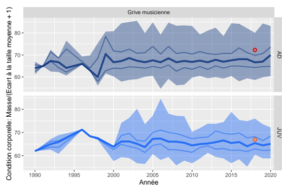
Figure 45: Variation de la condition corporelle des Grive musicienne pour le station 12 comparée aux STOC-Capture de type terrestre (n=230)
