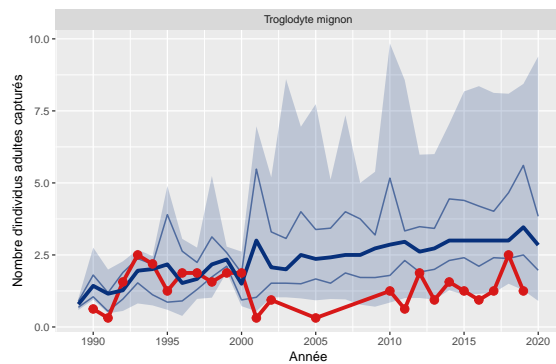
Figure 13: Variation du nombre d'adultes capturés de Troglydte mignon pour le station 12 comparé aux STOC-Capture de type terrestre (n=230)
